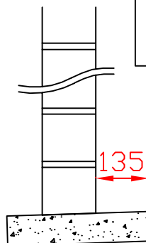
Schuifraam monorail met muggenraam aan binnenzijde
