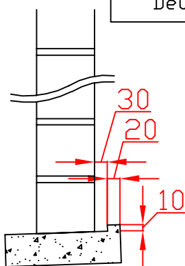
Schuifraam zonder rolluik
